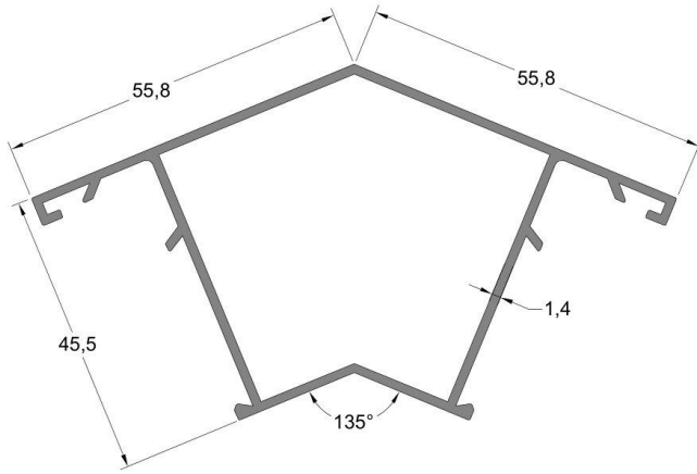
135° Köşe Dönüş Profili 135° CORNER PROFILE Profil Kodu Profile Code (kg/mt) Weight 160 0,872
