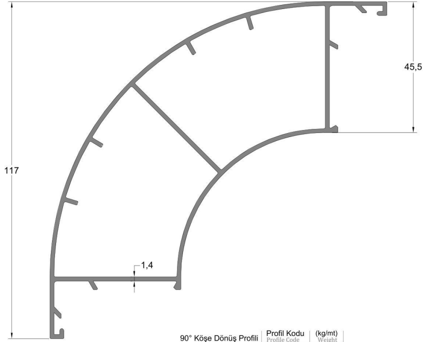
90° Köşe Dönüş Profili 90° CORNER PROFILE Profil Kodu Profile Code (kg/mt) Weight 404 1,728
