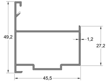
Pivot Adaptör Profili PIVOT ADAPTER PROFILE Profil Kodu Profile Code (kg/mt) Weight 7397 0,590
