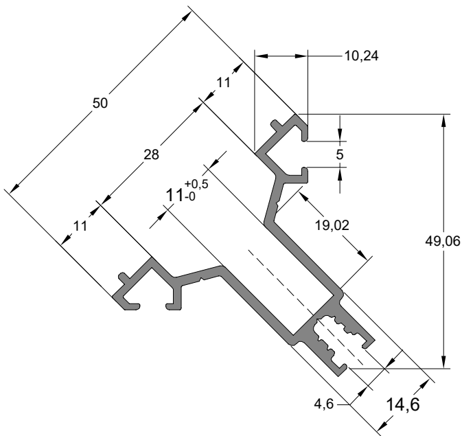
90° Dıştan Köşe Dönüş Profili 90° CORNER COVER PROFILE
