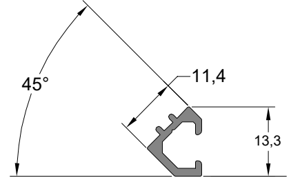
90° Dıştan Dönüş Çıta Profili 90° CORNER BEAD PROFILE
