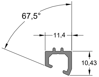
135° Köşe Dönüş Çıta Profili 135° CORNER BEAD PROFILE
