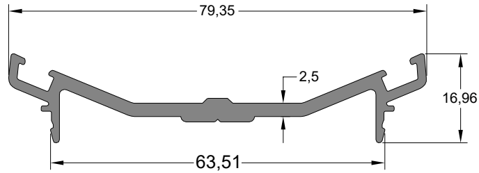
135° Köşe Dönüş Baskı Profili 135° CORNER EXTENSION PROFILE
