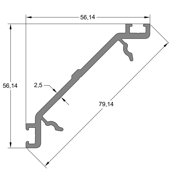
90° İçten Köşe Dönüş Profili 90° CORNER COVER PROFILE
