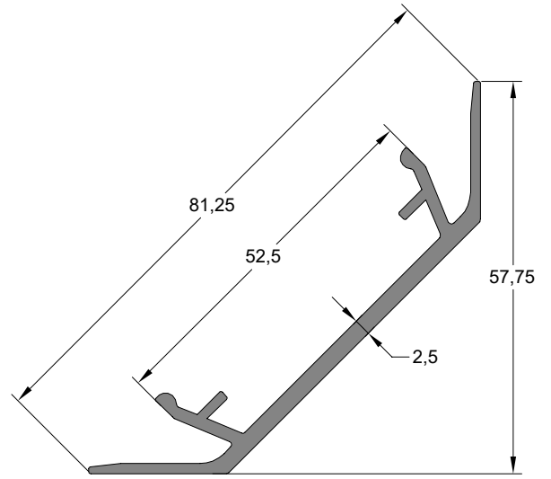
90° İçten Köşe Dönüş Profili 90° CORNER COVER PROFILE
