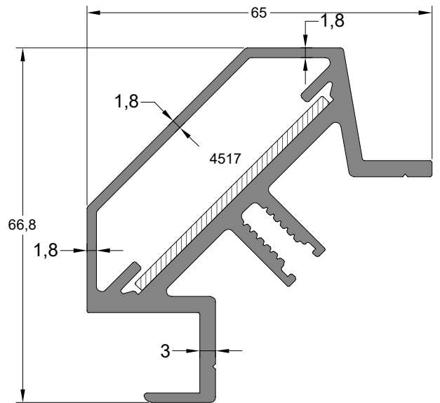
90° İçten Köşe Dönüş Profili 90° CORNER COVER PROFILE
