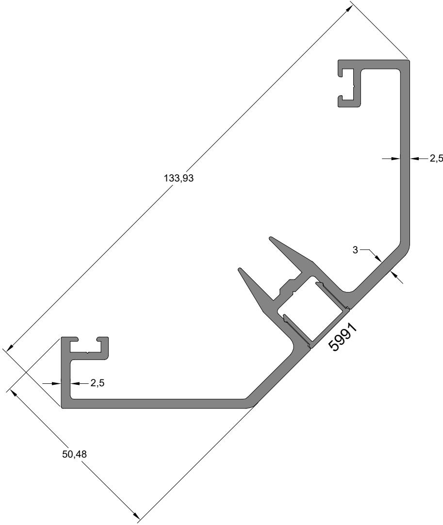
90° Dıştan Köşe Dönüş Kapak Profili 90° CORNER COVER PROFILE
