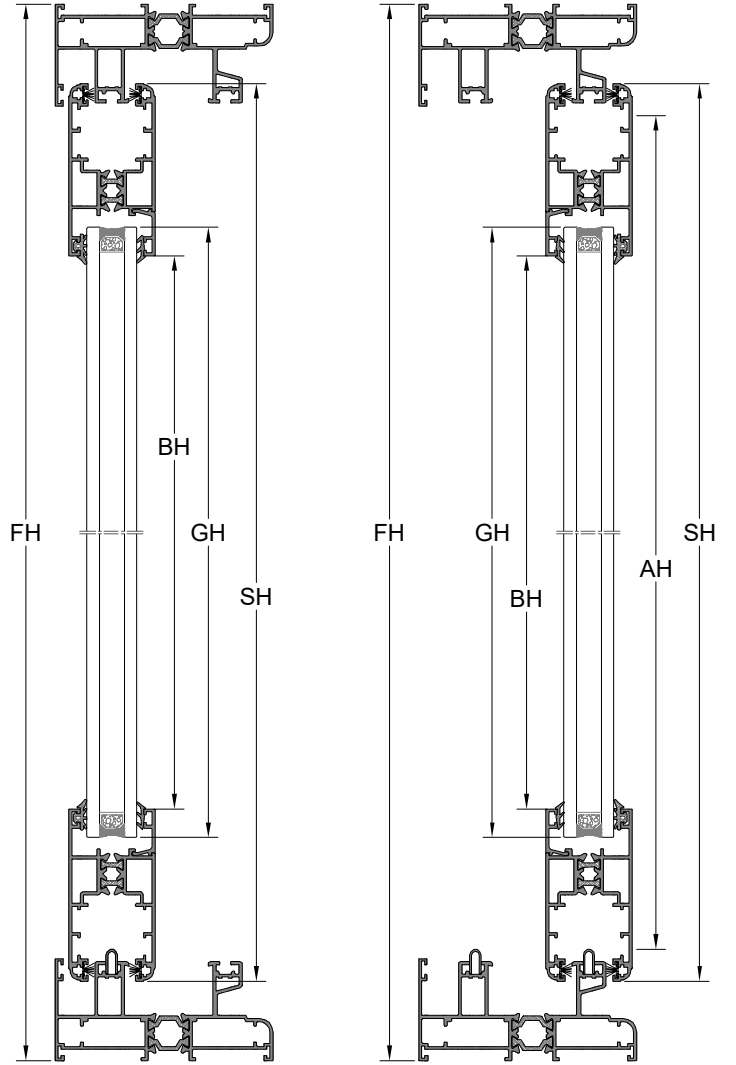
B-B KESİTİ
