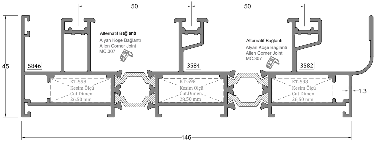
Üç Raylı Sineklikli Kasa Profili TRIPLE RAIL SCREENING FRAME PROFILE
