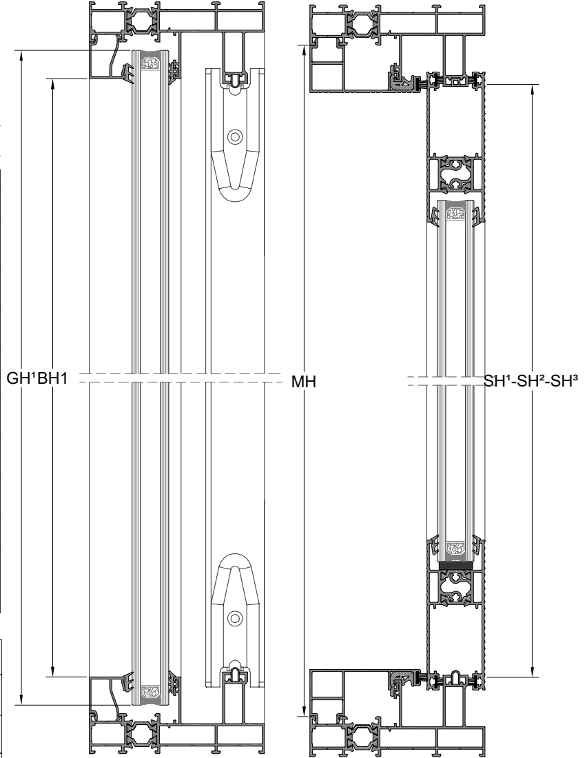
C-C KESİTİ
