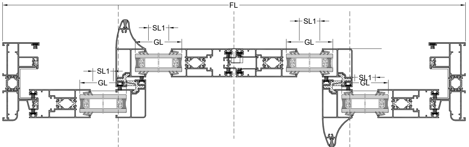
A-A KESİTİ
