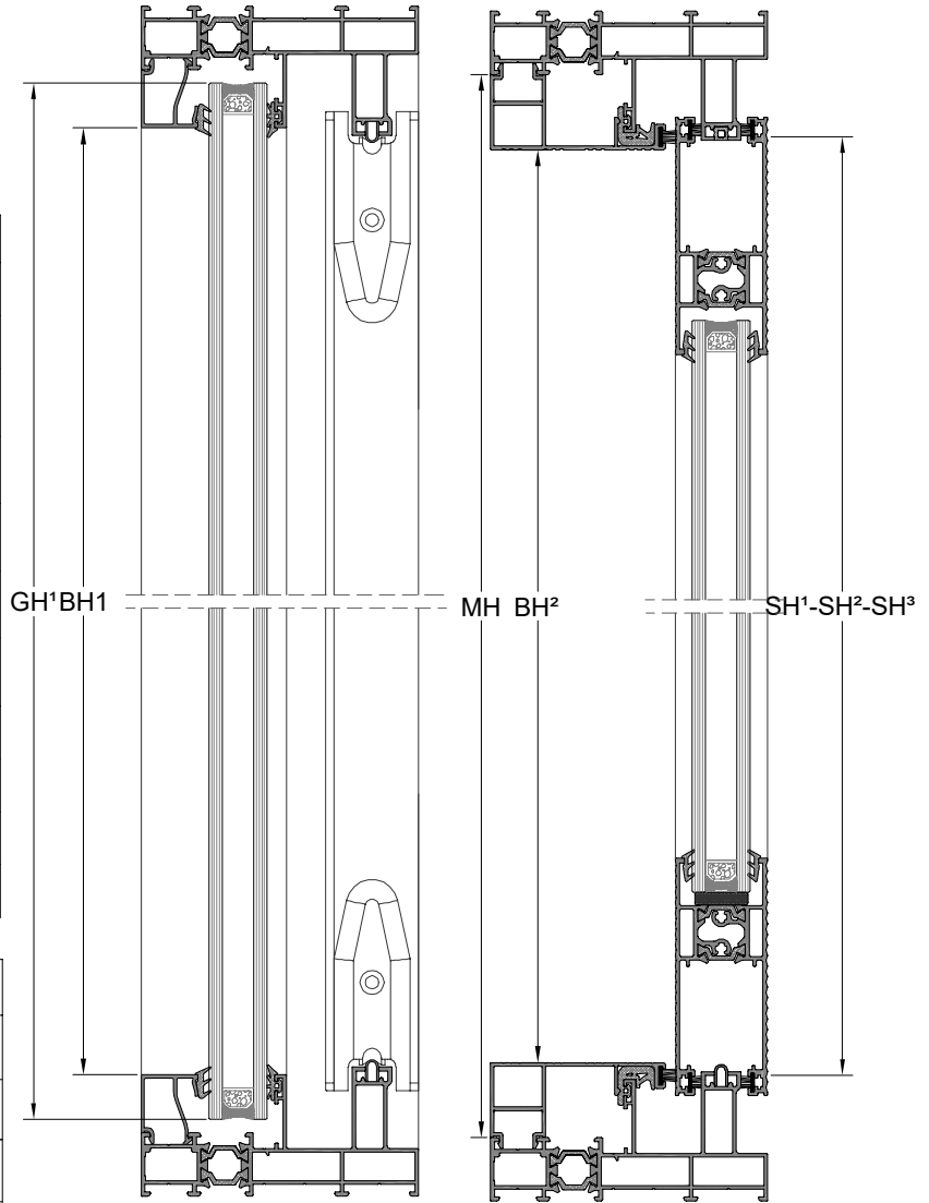
C-C KESİTİ
