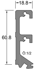
Orta Kayıt Bağlantı Profili MULLION CONNECTION PROFILE Profil Kodu Profile Code (kg/mt) Weight 11626 1,502
