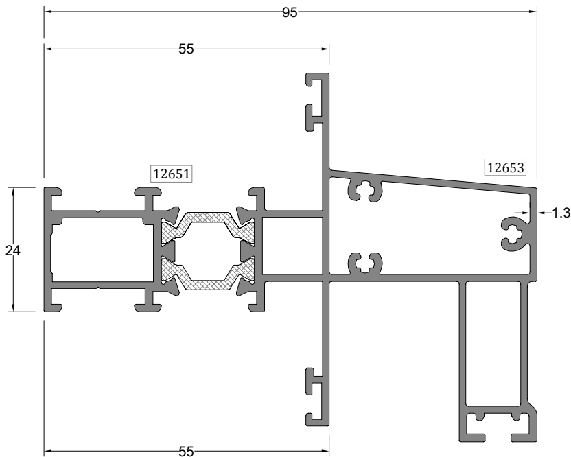
Sabite Geçiş Profili ADAPTER TO FIXED FRAME
