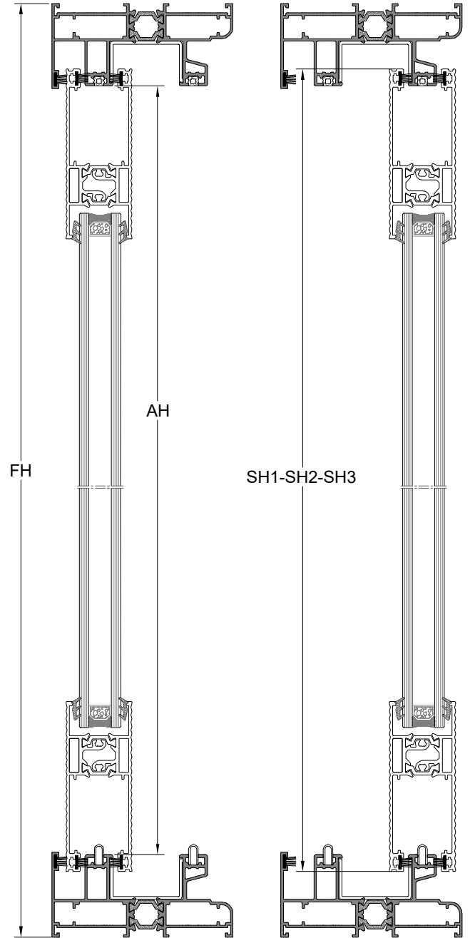
B-B KESİTİ
