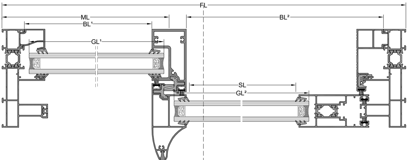
A-A KESİTİ
